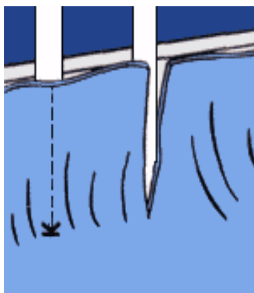
Рис.2.14. Укладання лінолеуму навколо труб
