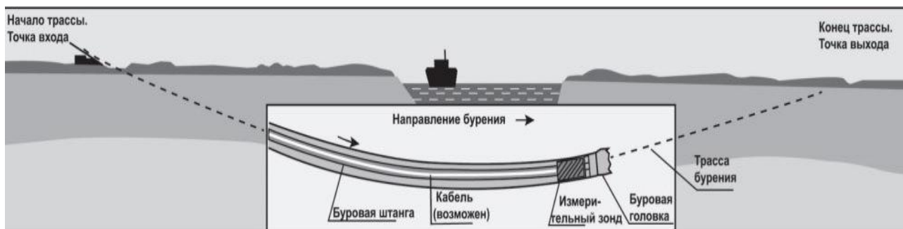
Рис. 3.3. Спрямоване буріння пілотної свердловини
