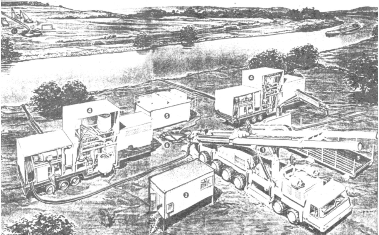
Рис. 3.2. Схема розміщення обладнання на будівельному майданчику при ГНБ:
